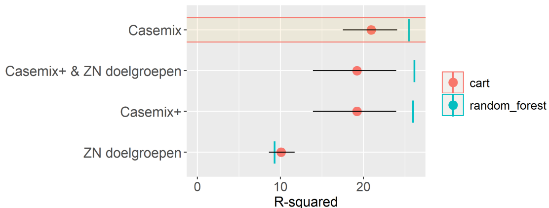
Figuur 11: CART en random forest resultaten (formele uren)
