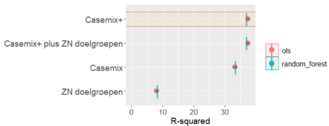
Figuur 24: Regressie (ols) en random forest resultaten (formeel en informele uren)
