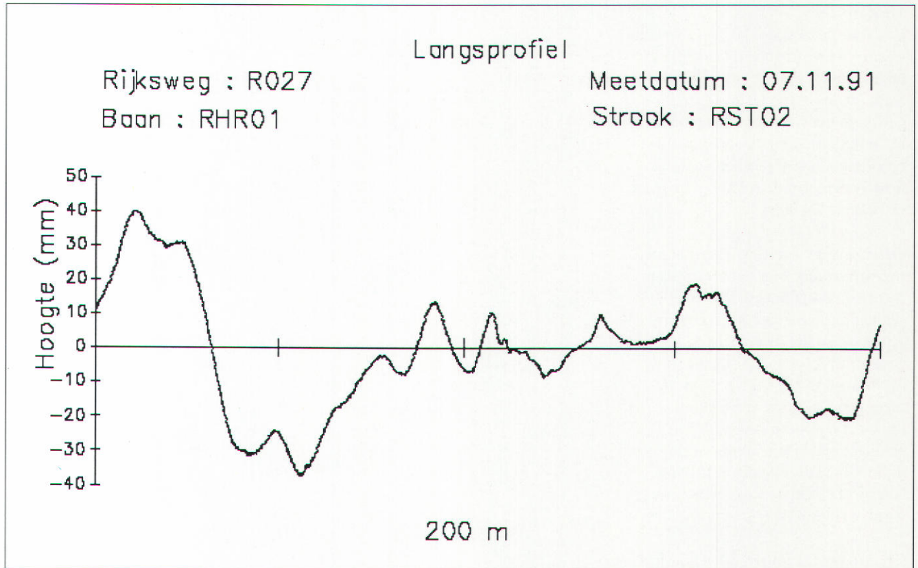
Figuur 3: Langsprofiel ARAN
