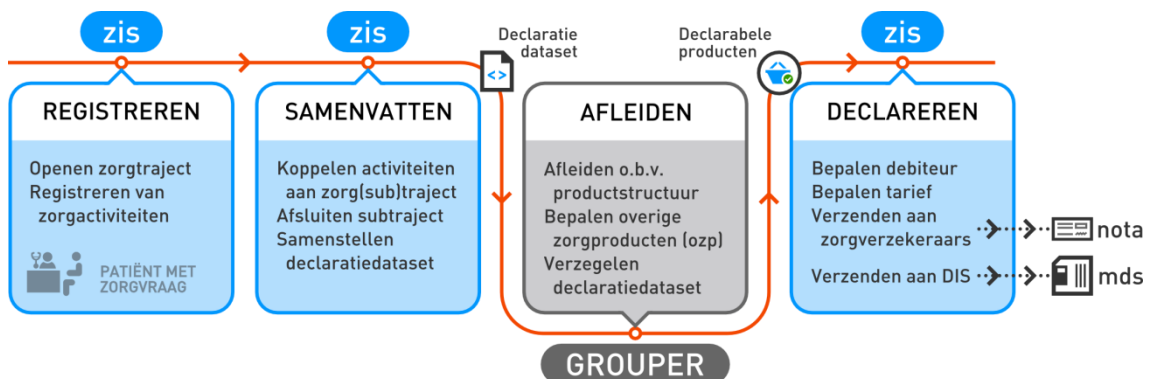
Figuur 4 RSAD-datamodel
