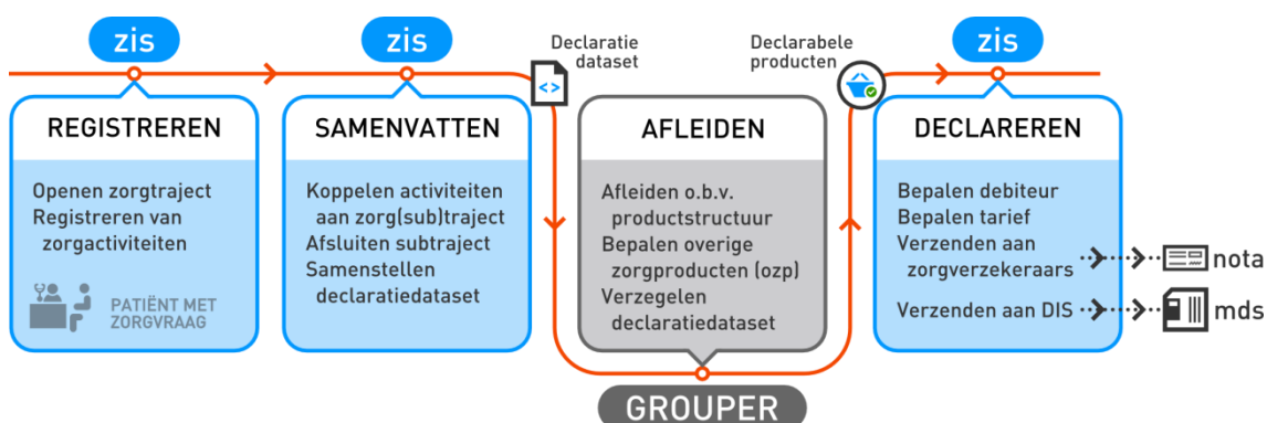
Figuur 4 Conceptueel RSAD-model
