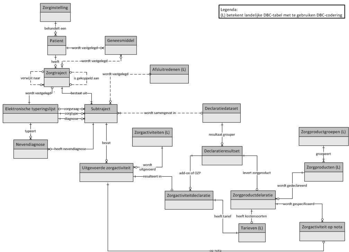
Figuur 15 RSAD-datamodel
