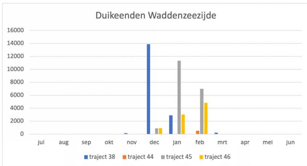
Figuur 6.4 Verdeling van de gemiddelde aantallen bodemdieretende duikeenden (= toppereenden) per maand in teltrajecten 38, 44, 45 en 46 (Waddenzeezijde) in de periode 2016/2017 – 2020/2021 (bron: maandelijkse vliegtuigtellingen Rijkswaterstaat en Sovon).
