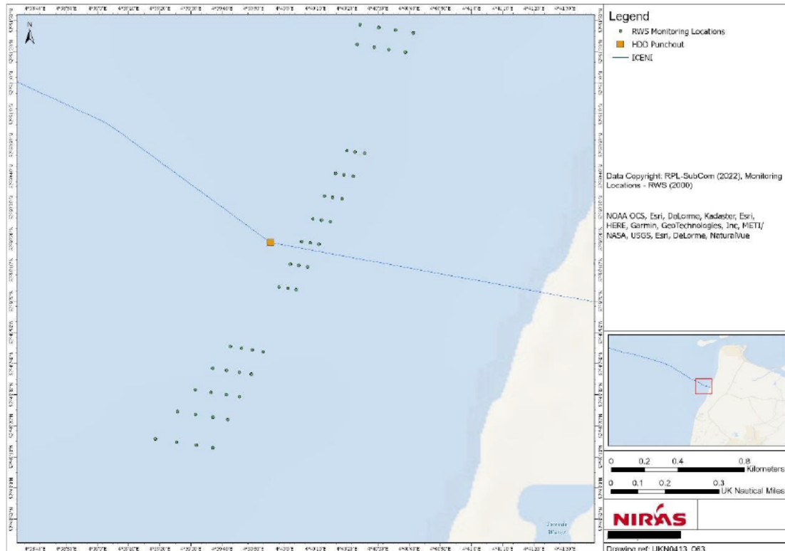
Figuur 2.3b Ligging HDD uitredepunt ten opzichte van monitoringpunten RWS
