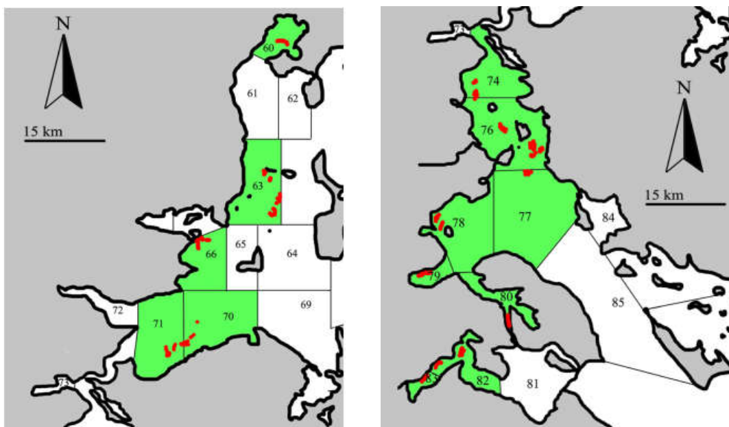
Figuur 2: De locaties van de monsternames Inags de North East Coast van Jutland (links) en langs de South East coast van Jutland (rechts). De nummers van de deelgebieden zoals weergegeven in figuur 2 komen overeen met de nummers zoals deze door de Deense overheid gehanteerd worden bij de monitoring op toxines en toxische algen in schelpdiergebieden.
