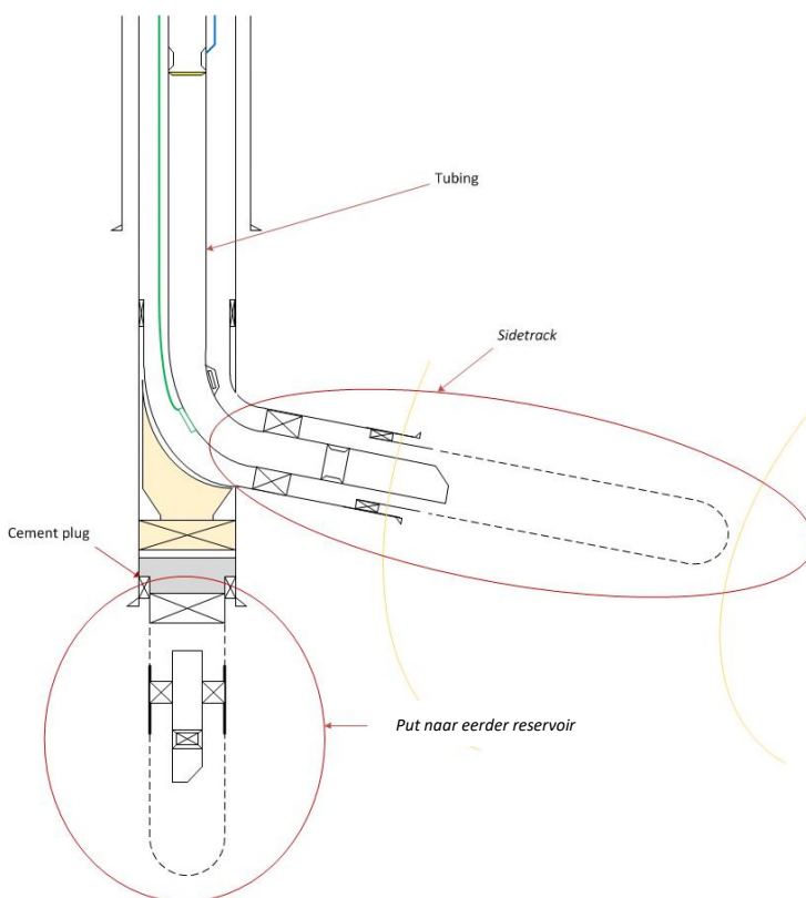
Figuur 3.3: Schematische afbeelding van een "sidetrack" boring
