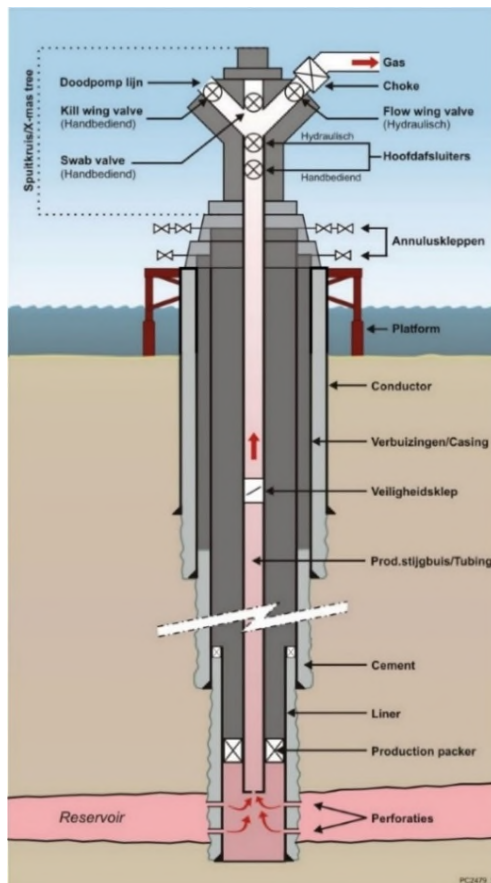
Figuur 3.4: Schematische afbeelding van een boorgat met verbuizingen
