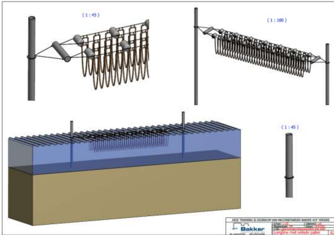
Figuur 7: schematische weergave van de mosselhangcultuur met paalankers
